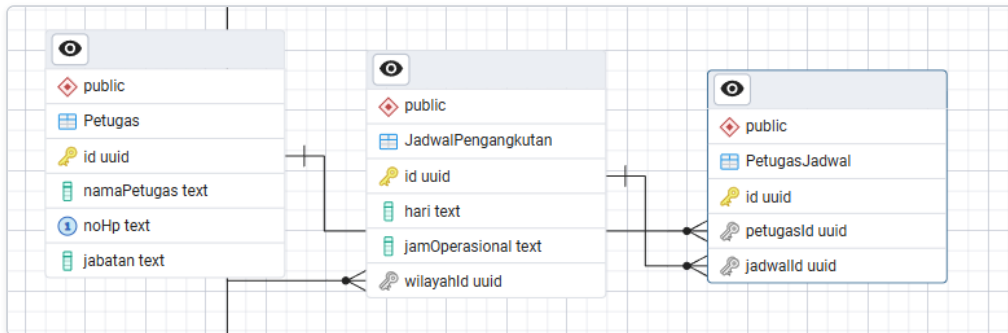
Gambar 11. Diagram Relasi Many-to-Many (N:N) pada pgAdmin
