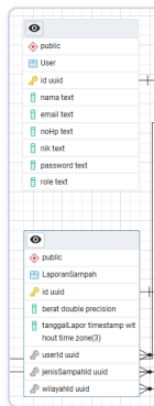
Gambar 10. Diagram Relasi One-to-Many (1:N) pada pgAdmin
